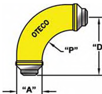
90° Long Sweep Ell (LSE90)
